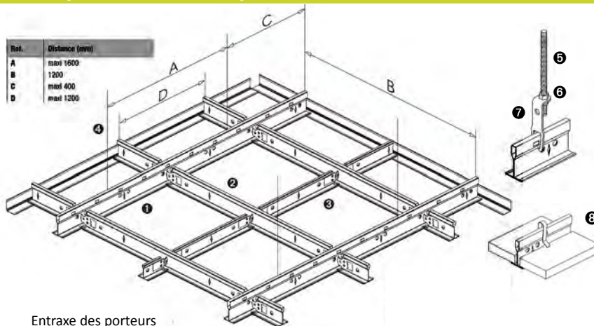
Entraxe des porteurs
