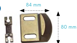
Guide fermeture
