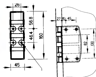
Charnière 4521 composite avec arrêt à 90°
