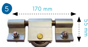
Galet mobile 3340
