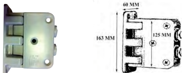
Charnière 1519 avec arrêt à 90°
