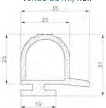
Mt Joint d'étanchéité périmétral Vendu au m., noir
