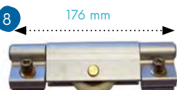
Galet mobile depuis 1996 Ø 50
