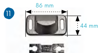
Guide fermeture 2120 / 2130
