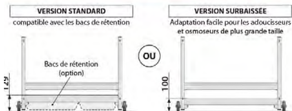
UN MODÈLE DE CHARIOT POUR DEUX CONFIGURATIONS
