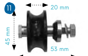
Galet et visserie 2320 avant 97
