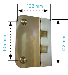
Charnière inox/polyamide arrêt à 90°
