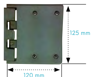
Charnière 3500
